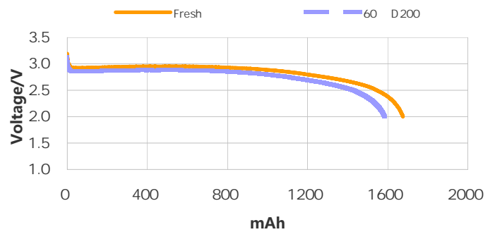
放电曲线 ( 20mA to 2.0V )
