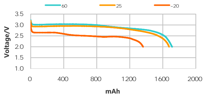
不同温度放电曲线 ( 20mA to 2.0V )
